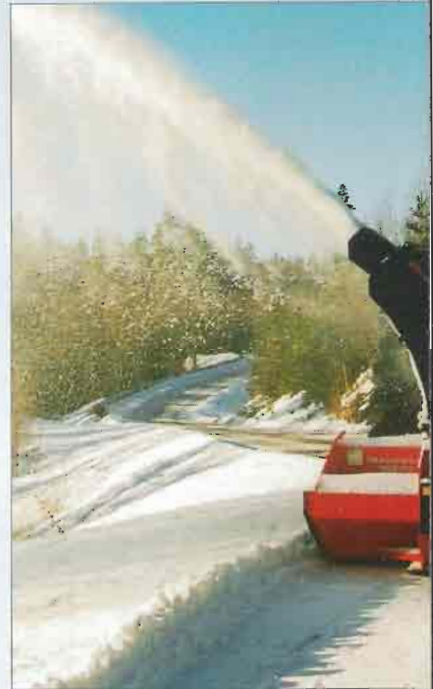
Die Schleppschuhe sind höhenverstellbar und die Verschleißleiste hat 2 Verschleißseiten.
